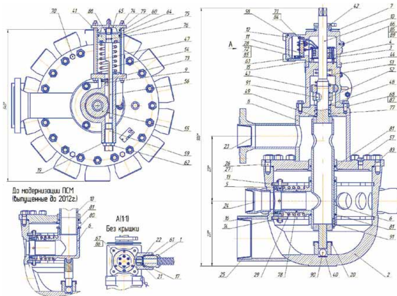
Общий вид PCM: Ха2.954.008; Ха2.954.034; PCM12.00.00.000
